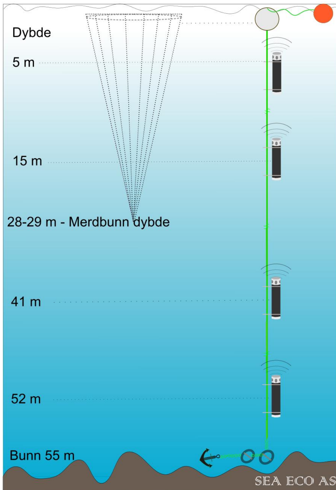
Fig. 34 Prinsippskisse for riggoppsett av strømmålere. Målingene som er rapportert er fra 5 m, 15 m, 41 m og 52 m dyp. Merdbunn er beregnet ut fra posetype, spisspose 28-29 m. Bunndyp ca. 55 m.
