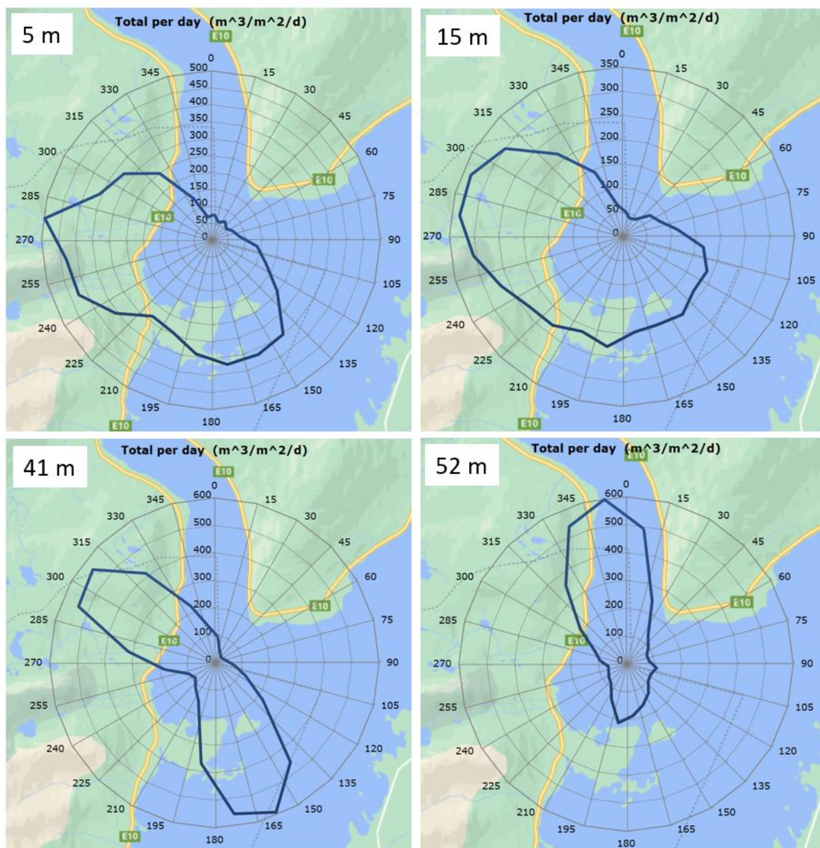
Fig. 19 Vannforflytning (m 3 /m 2 /dag) på 5 m, 15 m, 41 m og 52 m dyp i løpet av 04.08.2022 – 03.10.2022. Grafen viser gjennomsnittlig vannforflytning per dag i forhold til retningsgrader .
