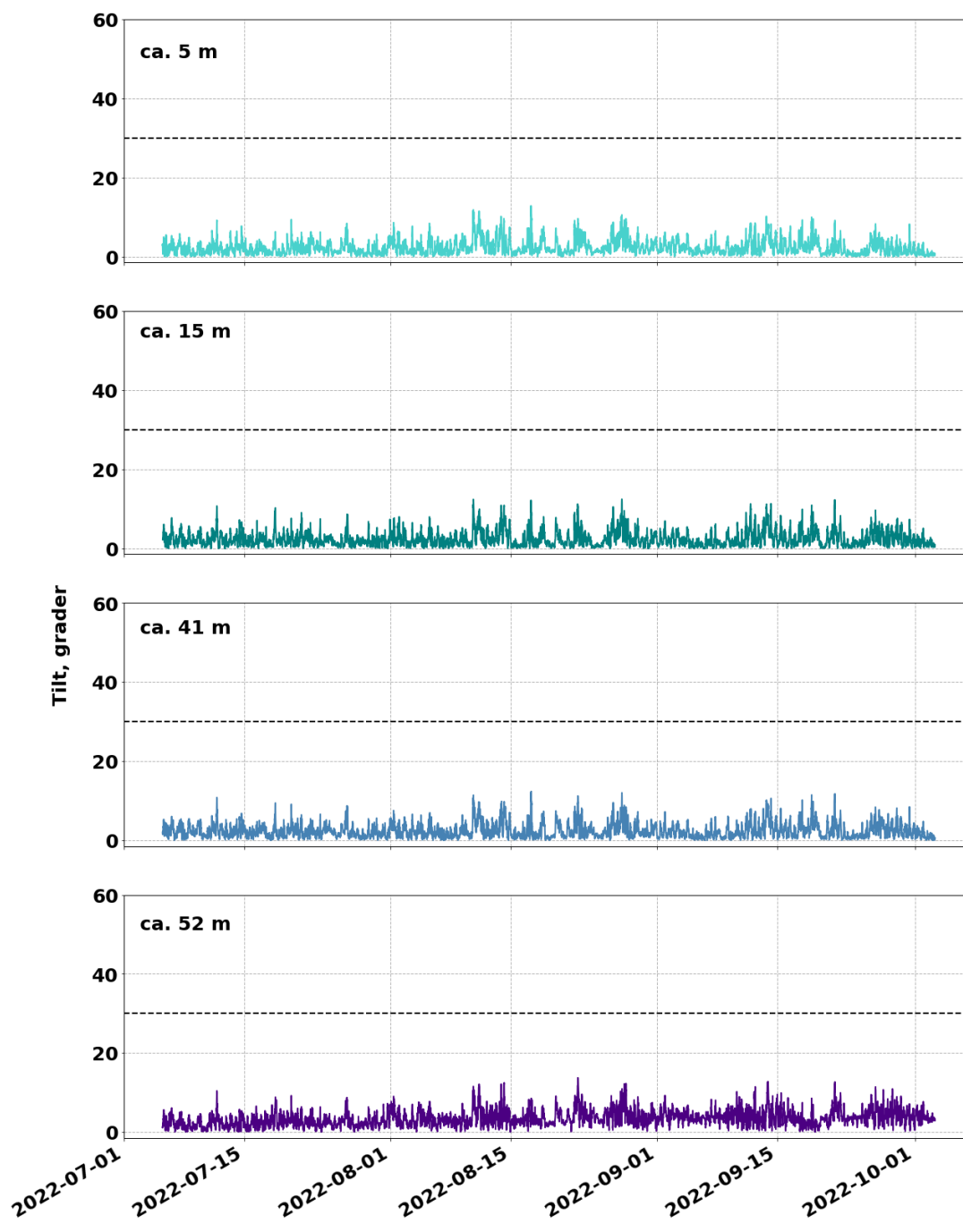
Fig. 32 Tilt (°) på 5 (turkis linje), 15 (mørk grønn linje), 41 (blå linje) og 52 m (fiolett linje). Stiplet linje indikerer 30° som er grenseverdien for høy tilt.
