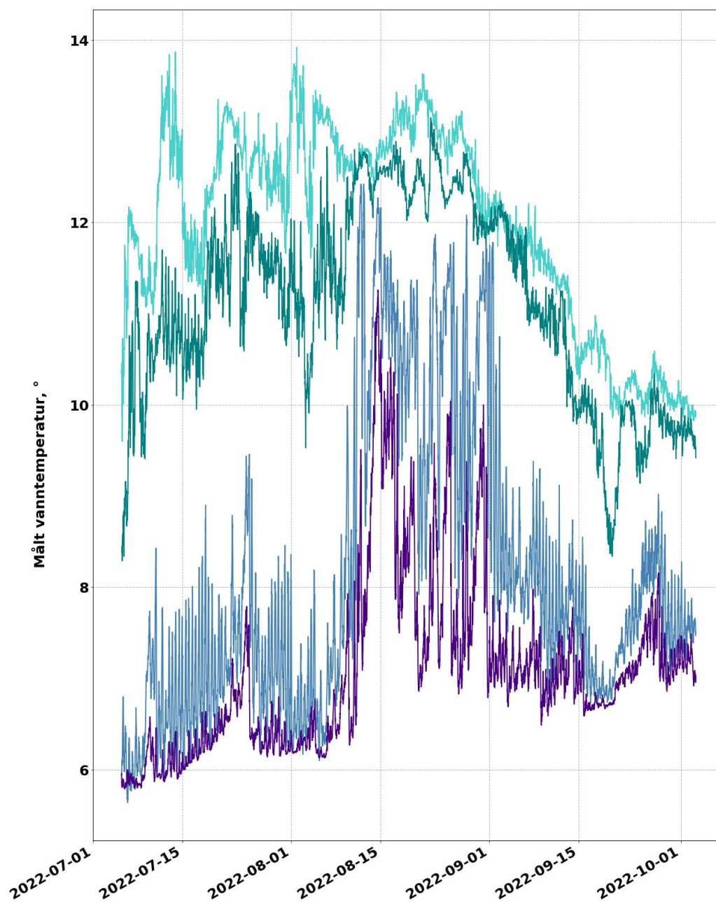
Fig. 28 Sjøtemperatur i løpet av måleperioden på 5 m (turkis linje), 15 m (mørk grønn linje), 41 m (blå linje) og 52 m (fiolett linje).
