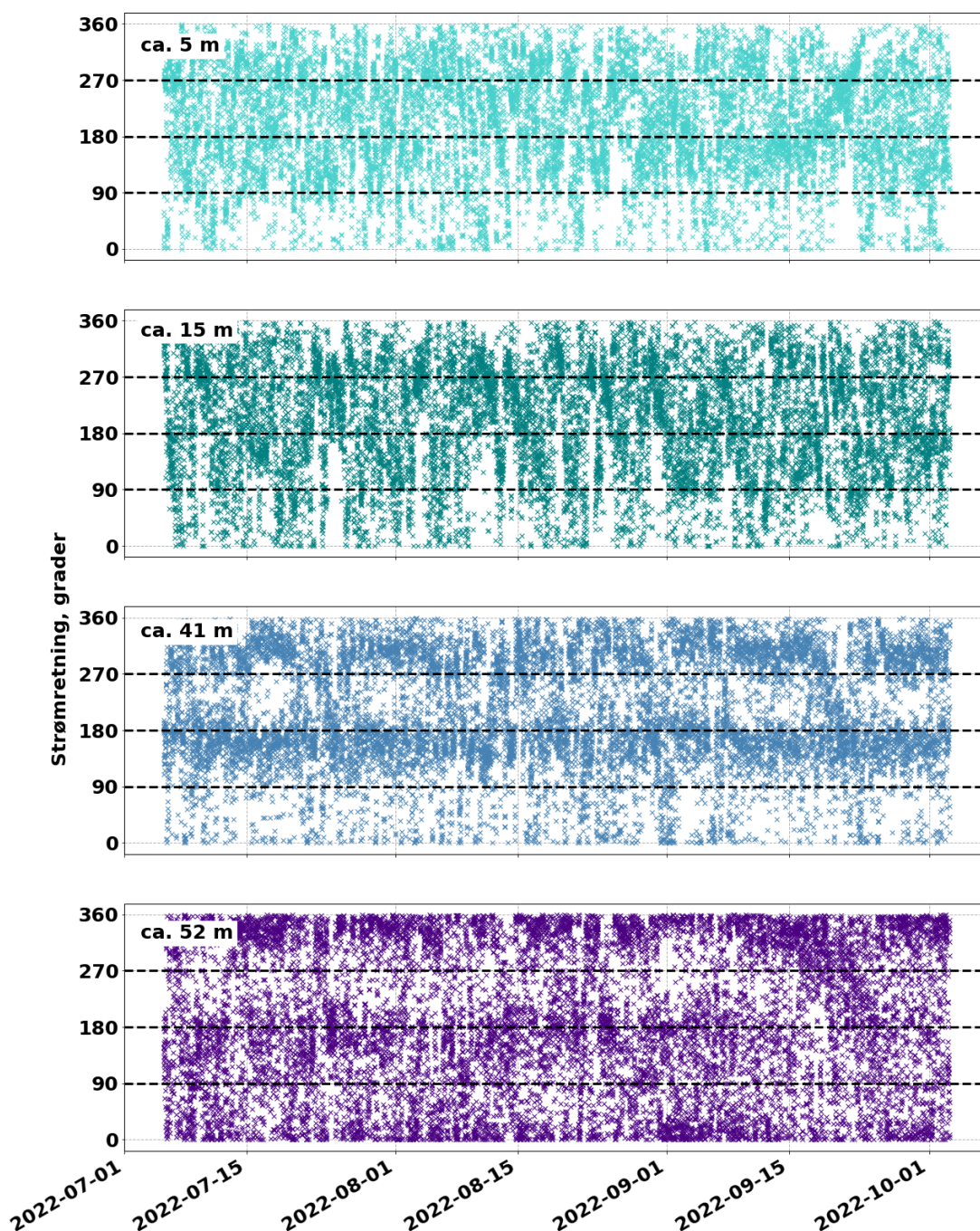
Fig. 6 Logget strømretning på 5 m (turkis farge), 15 m (mørk grønn farge), 41 m (blå farge) og 52 m (fiolett farge). De fleste målinger registrerte strømretninger mellom 247,5-292,5° (mot vest) på 5 og 15 m dyp. De fleste målinger registrerte strømretninger mellom 157,5-202,5° (mot sør) på 41 m dyp. De fleste målinger registrerte strømretninger mellom 337,5-22,5° (mot nord) på 52 m dyp.
