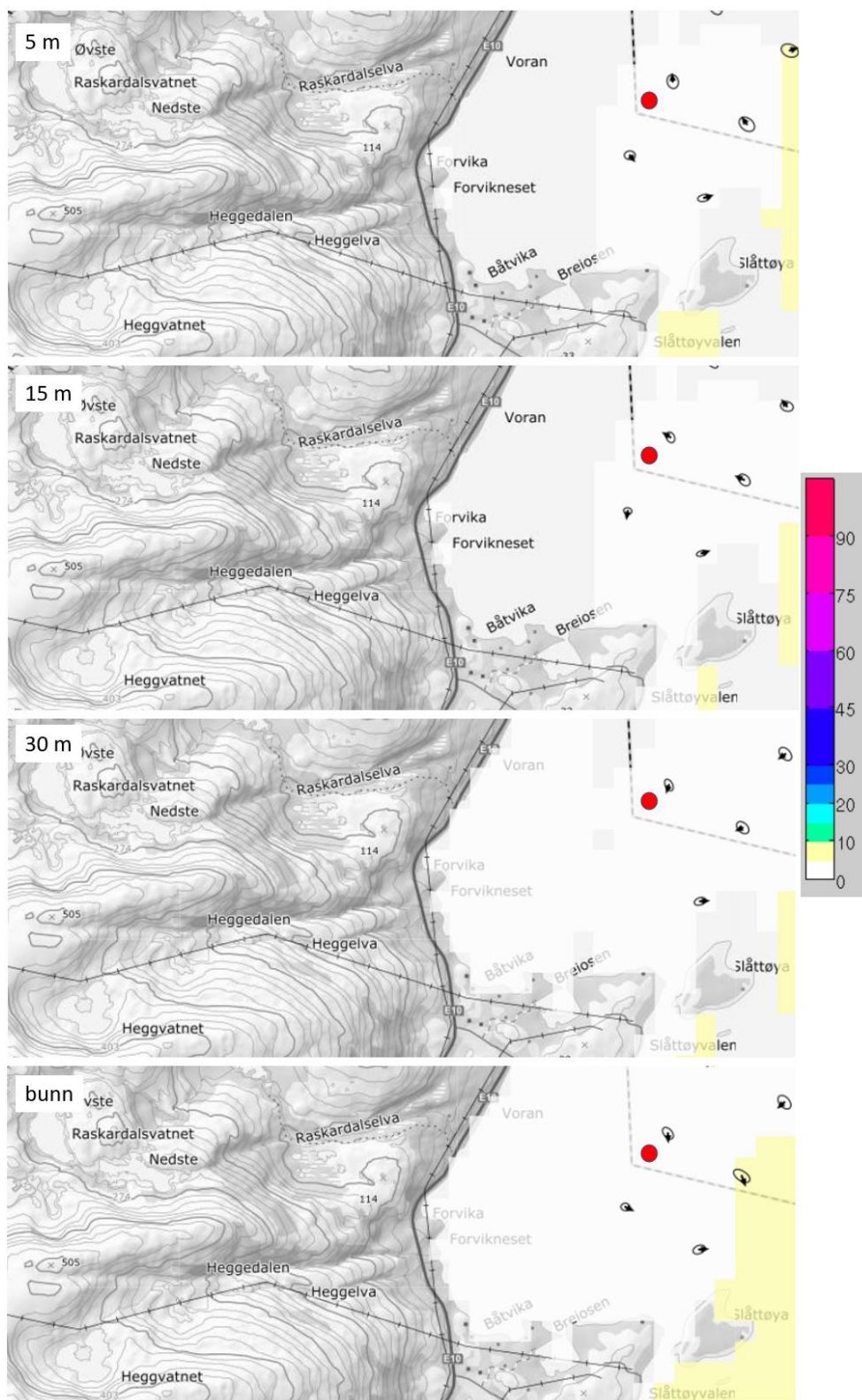
Fig. 21 - Havmodellingsverdier for 5 m, 15 m, 30 m dyp og bunn (årlig median 50. persentil) av strømshastighet i Lavangen (Havstraum:2022).
