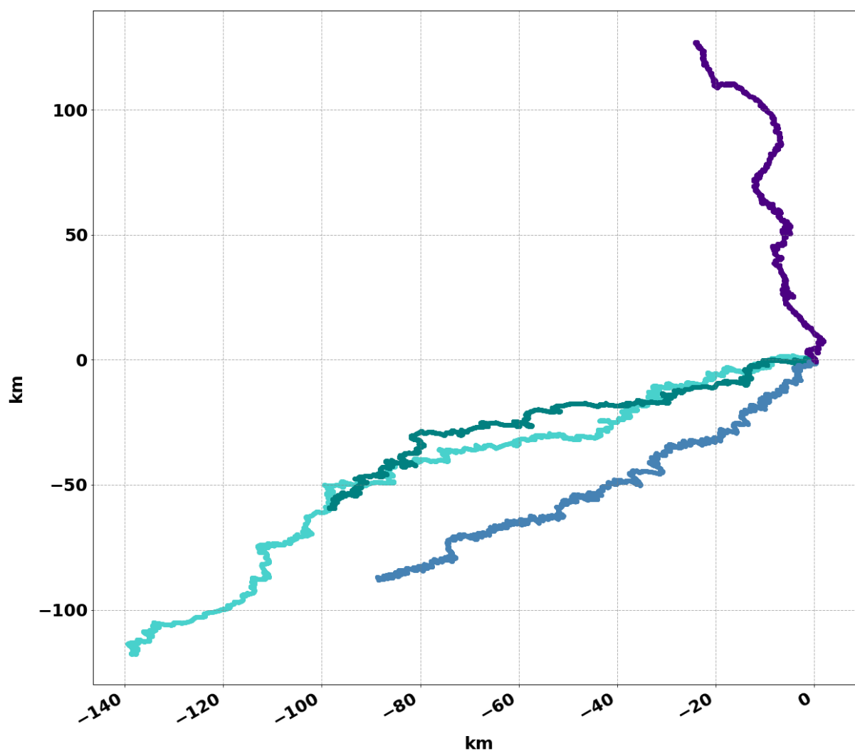
Fig. 17 Progressiv vektordiagram på 5 m (turkis linje), 15 m (mørk grønn linje), 41 m (blå linje) og 52 m (fiolett linje). Diagrammet sammenstiller strømstyrke, retning, tid og beregnet distanse for å vise flytting av vannpartiklene i måleperioden og gir et klart bilde av hovedstrømretningen. Denne er basert på en idealisert situasjon der målingene er gjort i åpent hav uten fysiske hindringer for strømmen.
