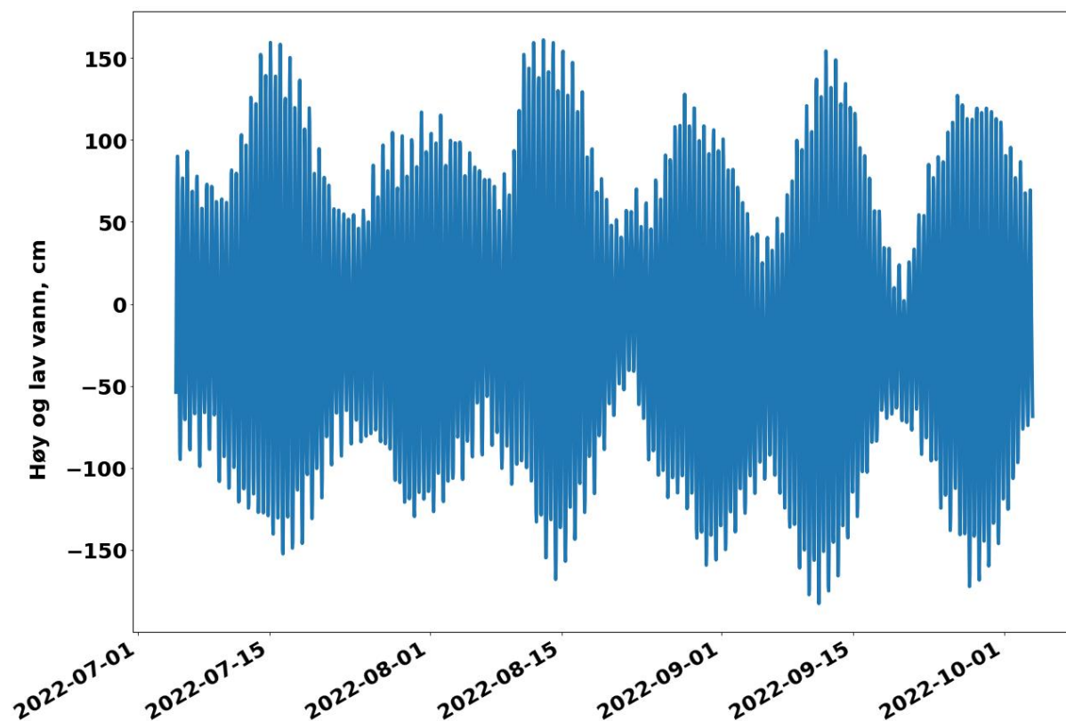
Fig. 22 Tidevann/høy- og lavvann ved Harstad målestasjon i perioden 05.07.2022 – 03.10.2022 (Kartverket, 2021).
