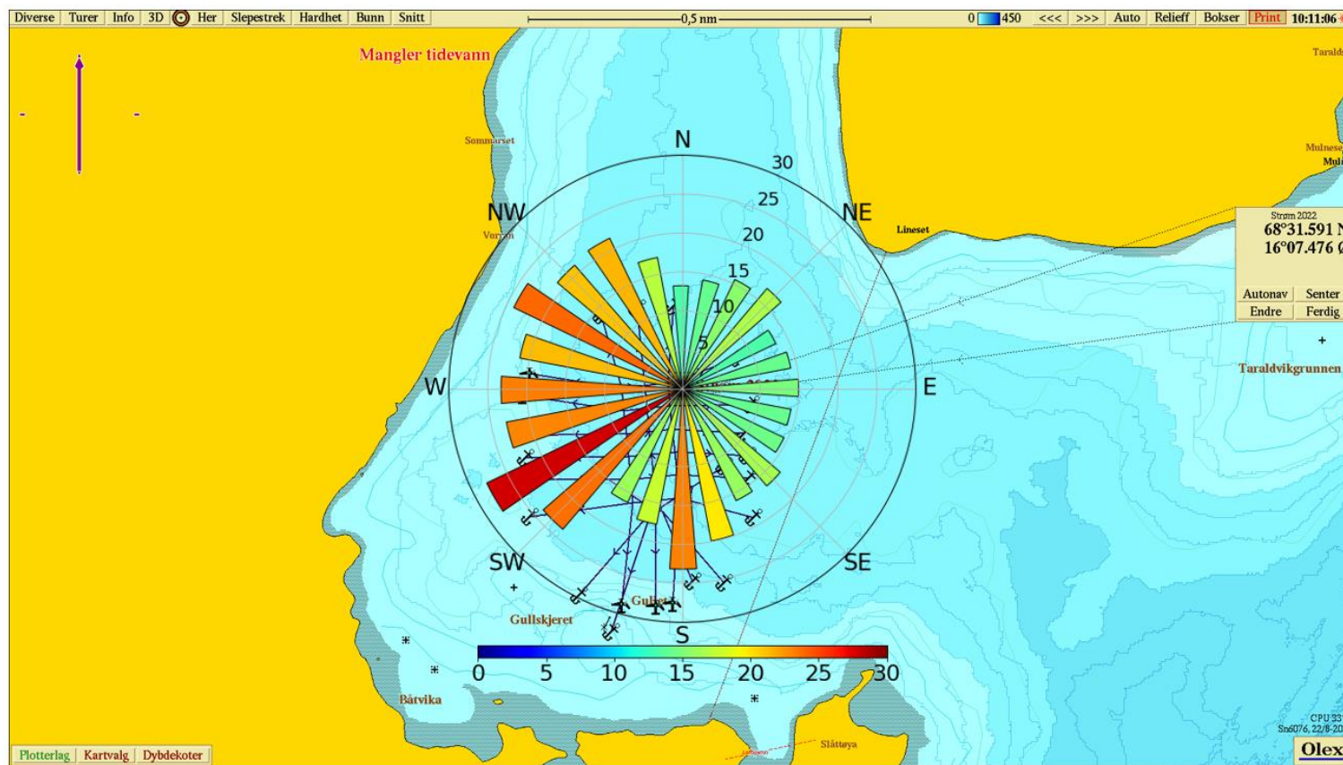
Fig. 11 Maks strømhastighet fremstilt som rosediagram (5 m) i Olex. Fargeskala fra 0 (mørk blå) til 30 cm/s (mørk rød).
