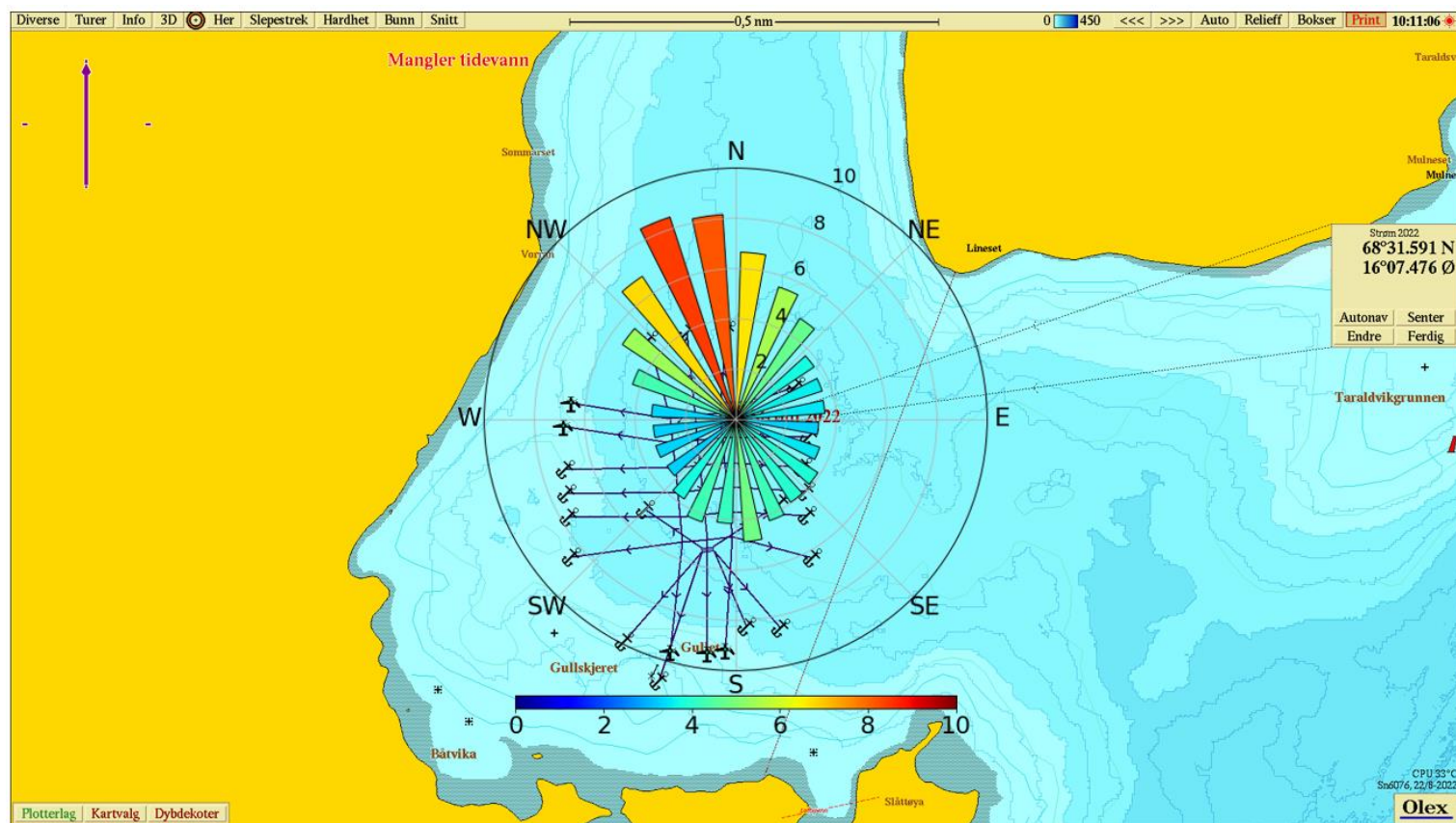
Fig. 10 Gjennomsnittlig strømshastighet fremstilt som rosediagram (52 m) i Olex. Fargeskala fra 0 (mørk blå) til 10 cm/s (mørk rød).
