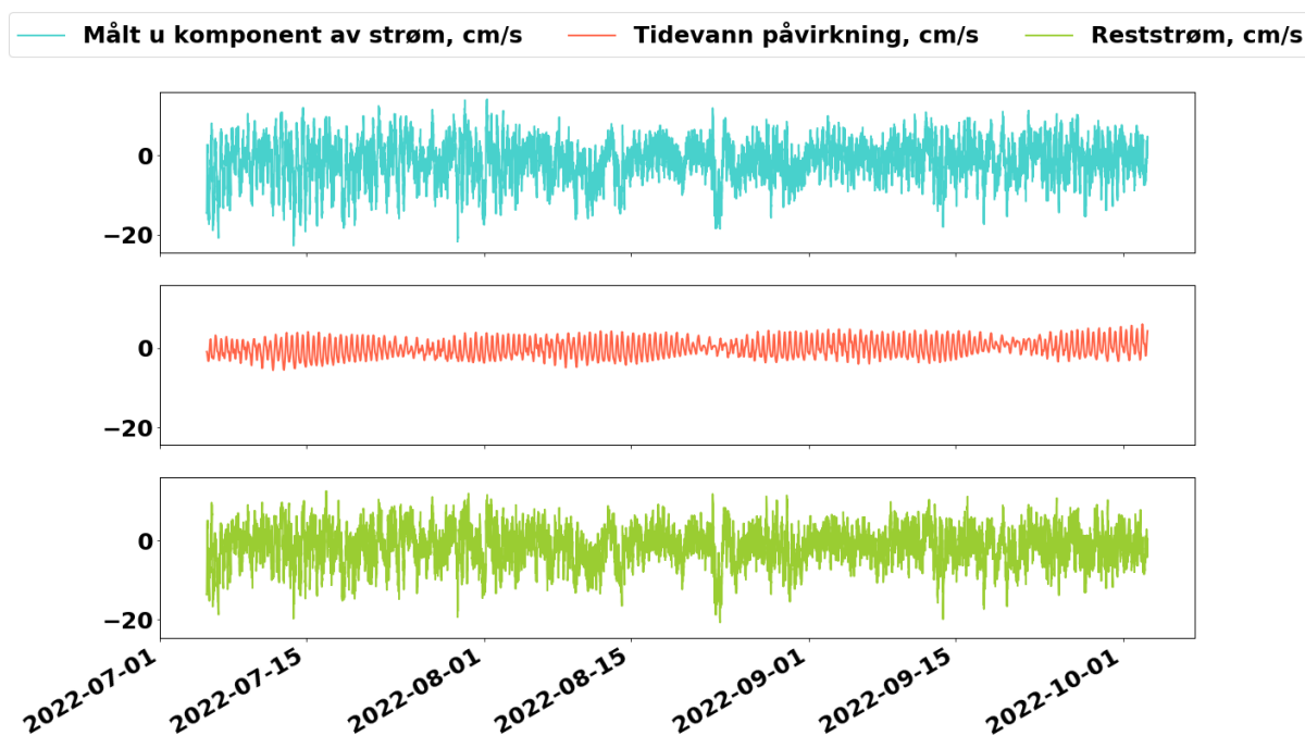
Fig. 26 Tidevannanalyse for strømshastighetsdata (cm/s) (u komponent på 5 m dybde) (UTide GSO Report:2011)
