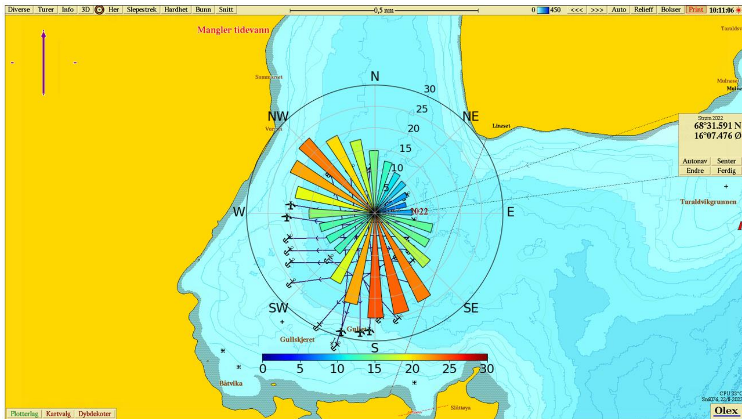
Fig. 13 Maks strømhastighet fremstilt som rosediagram (41 m) i Olex kart. Fargeskala fra 0 (mørk blå) til 30 cm/s (mørk rød).
