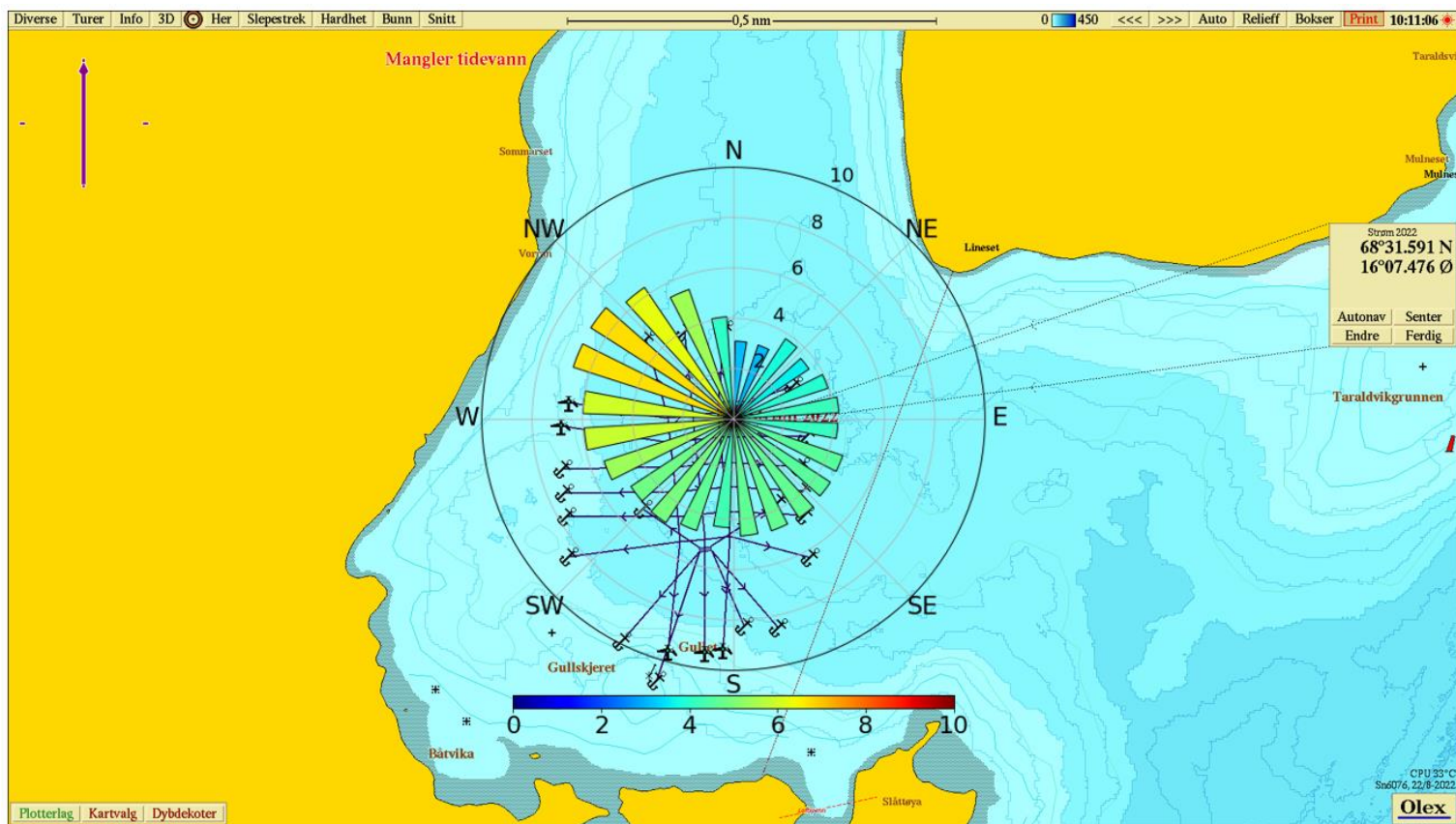
Fig. 8 Gjennomsnittlig strømhastighet fremstilt som rosediagram (15 m) i Olex. Fargeskala fra 0 (mørk blå) til 10 cm/s (mørk rød).
