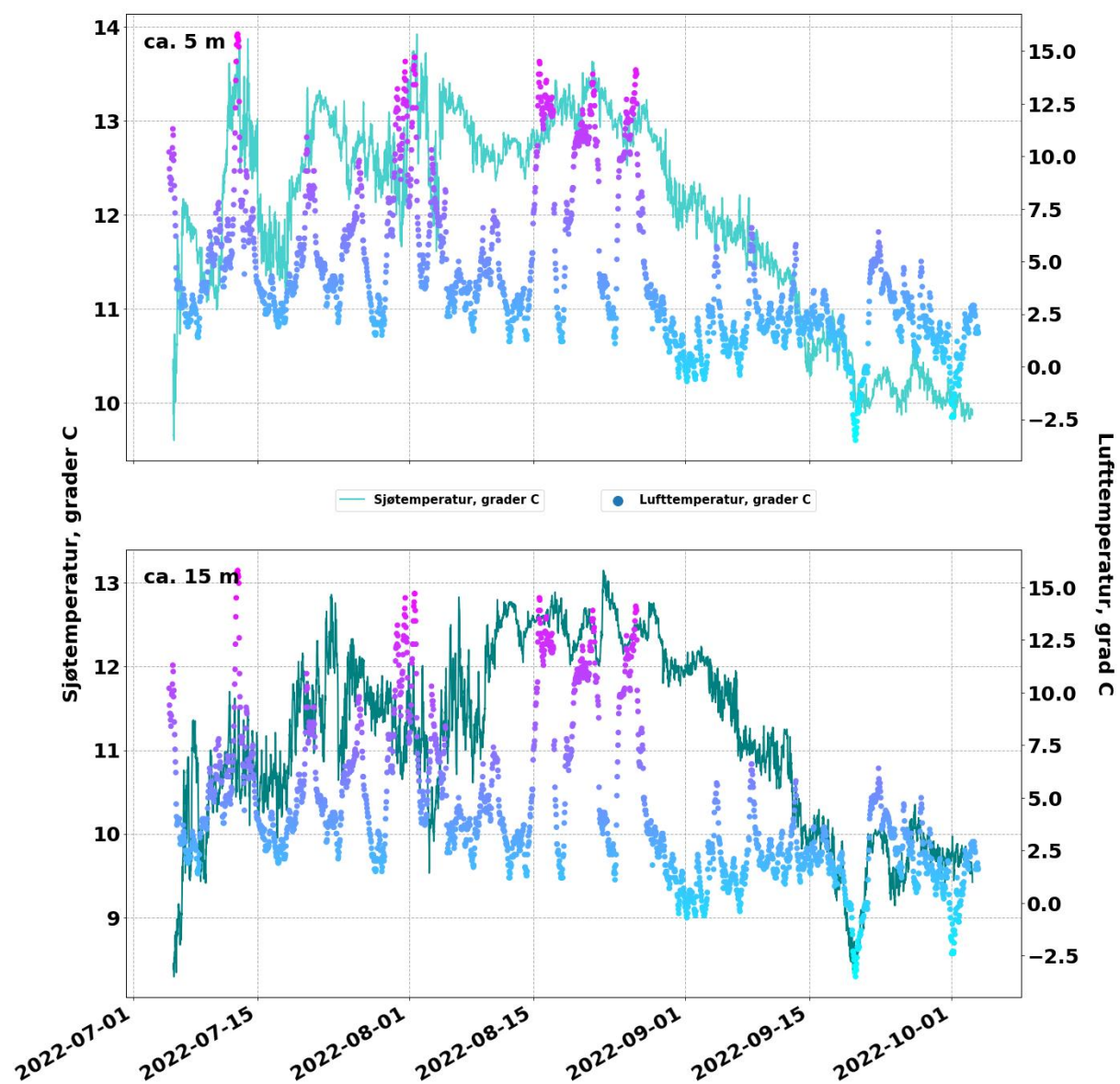
Fig. 30 Sjøtemperaturer på 5 m (øvre bilde) og på 15 m (nederste bilde) plottet i forhold til registrert lufttemperatur gjennom måleperioden (lufttemperatur data er hentet fra (SeKlima:2022))
