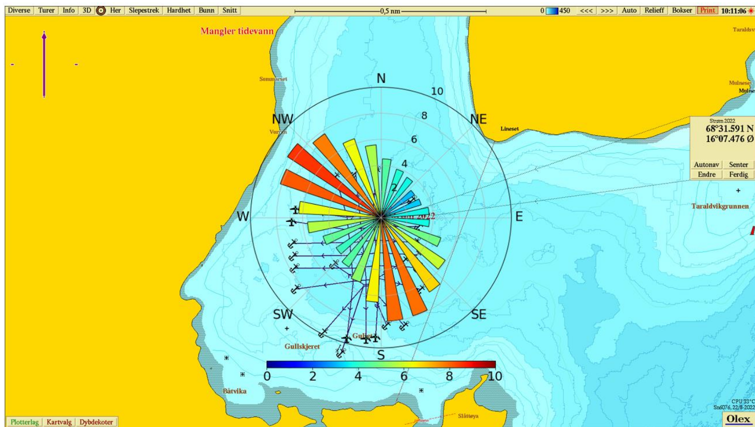
Fig. 9 Gjennomsnittlig strømhastighet fremstilt som rosediagram (41 m) i Olex. Fargeskala fra 0 (mørk blå) til 10 cm/s (mørk rød).
