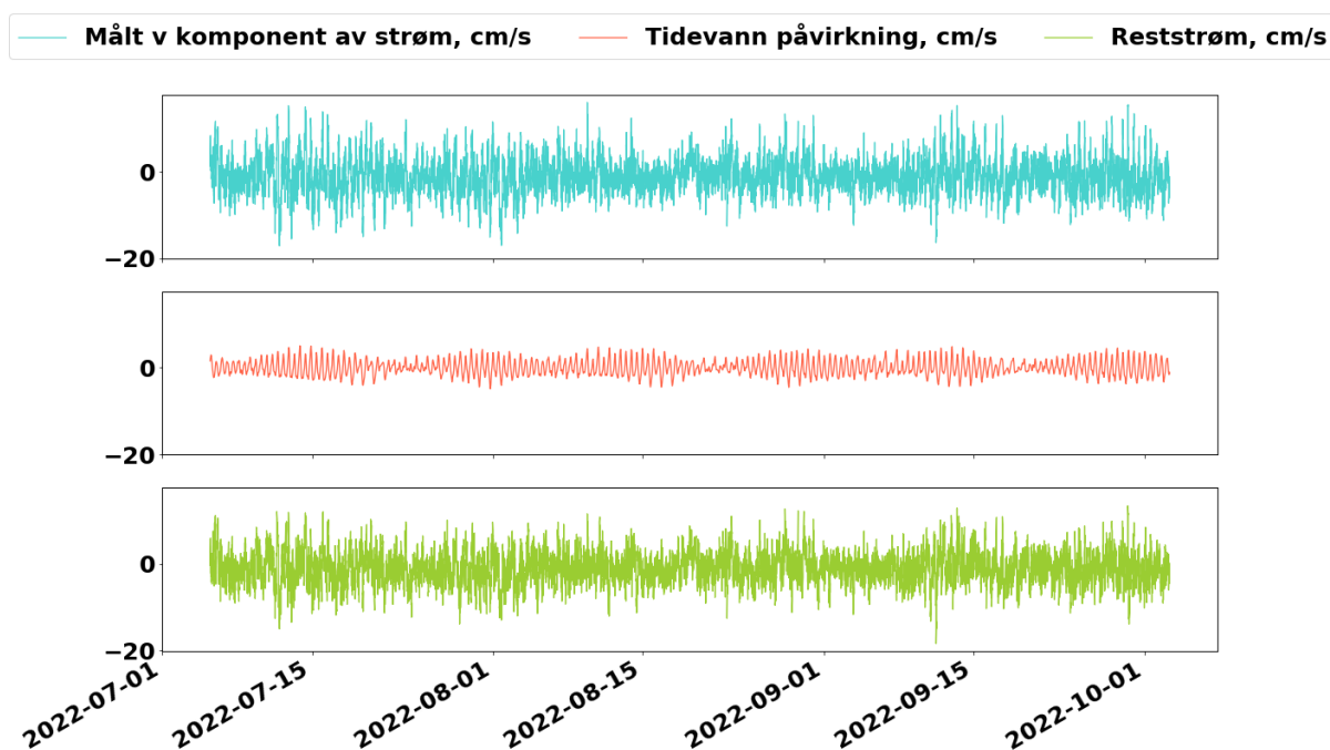
Fig. 27 Tidevannanalyse for strømshastighetsdata (cm/s) (v komponent på 5 m dybde) (UTide GSO Report:2011)
