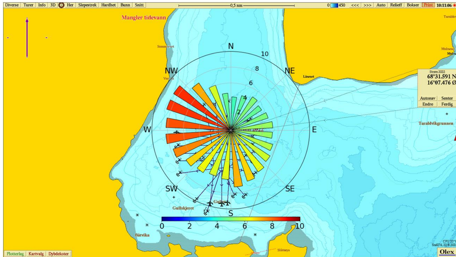
Fig. 7 Gjennomsnittlig strømhastighet fremstilt som rosediagram (5 m) i Olex. Fargeskala fra 0 (mørk blå) til 10 cm/s (mørk rød).
