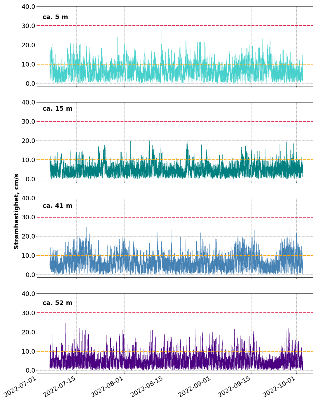
Fig. 5 Logget strømhastighet på 5 m (turkis linje), 15 m (mørk grønn linje), 41 m (blå linje) og 52 m (fiolett linje) dyp. Rød stiplet linje indikerer 30 cm/s som er grenseverdien for høy strømhastighet. Oransje stiplet linje er vist for forenklet visuell analyse av strømhastigheter over/under 10 cm/s.
