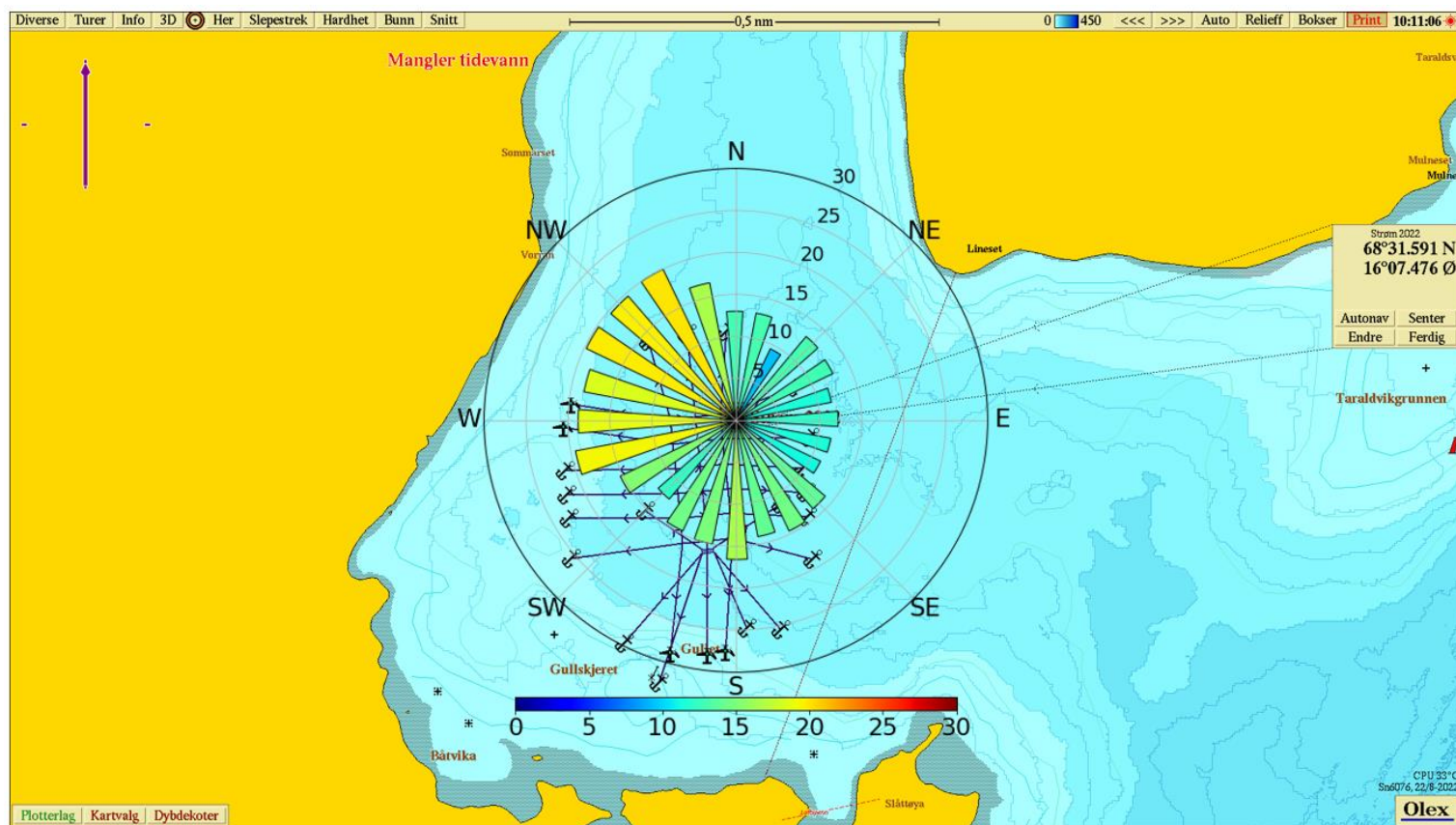
Fig. 12 Maks strømhastighet fremstilt som rosediagram (15 m) i Olex kart. Fargeskala fra 0 (mørk blå) til 30 cm/s (mørk rød).
