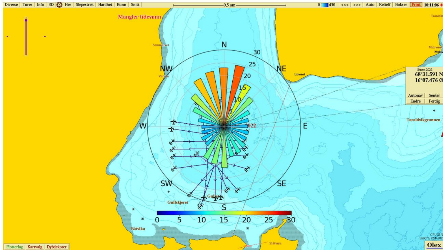
Fig. 14 Maks strømhastighet fremstilt som rosediagram (52 m) i Olex kart. Fargeskala fra 0 (mørk blå) til 30 cm/s (mørk rød).
