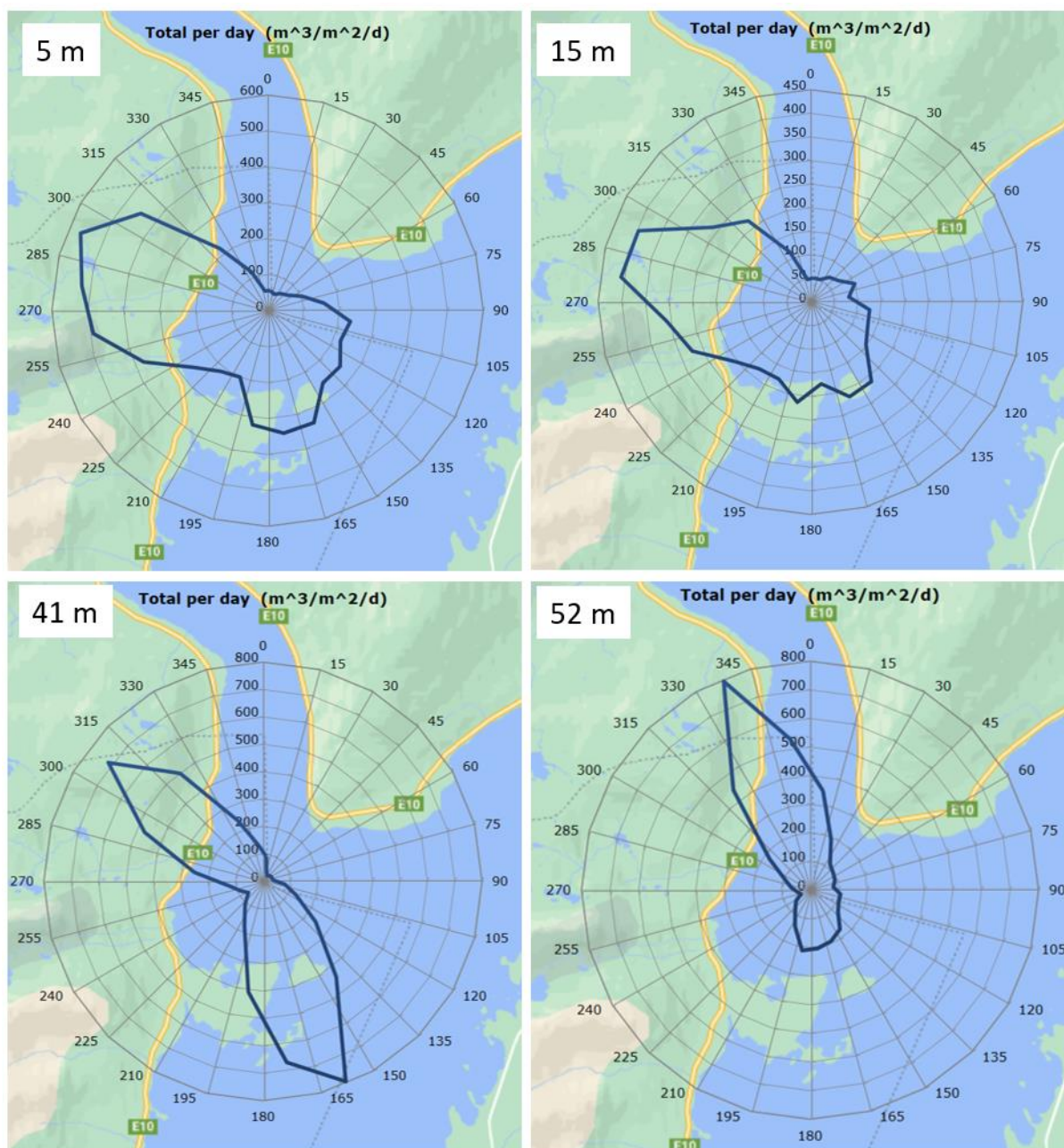
Fig. 18 Vannforflytning (m 3 /m 2 /dag) på 5 m, 15 m, 41 m og 52 m dyp i løpet av 05.07.2022 – 04.08.2022. Grafen viser gjennomsnittlig vannforflytning per dag i forhold til retningsgrader .
